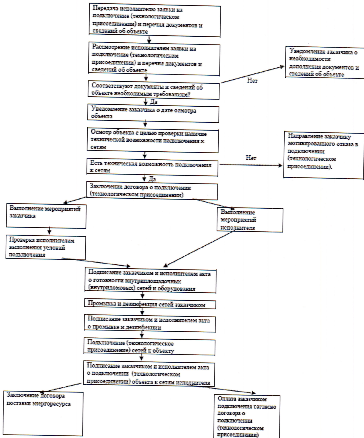
Блок-схема, отражающая графическое изображение последовательности действий, осуществляемых при подключении к централизованной системе холодного водоснабжения.
